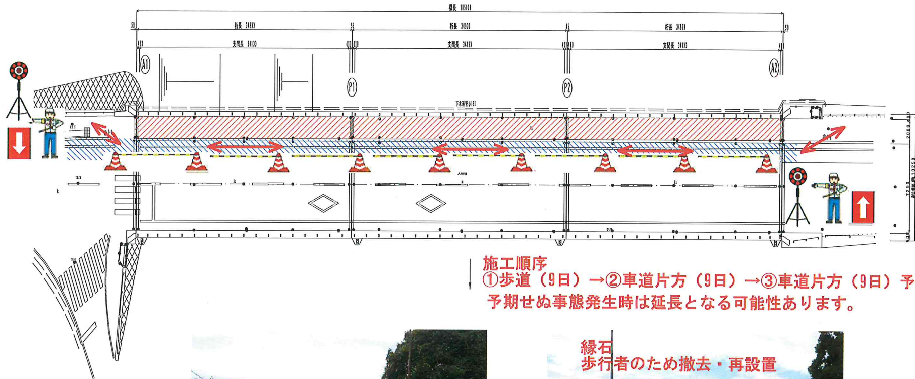
平面図
