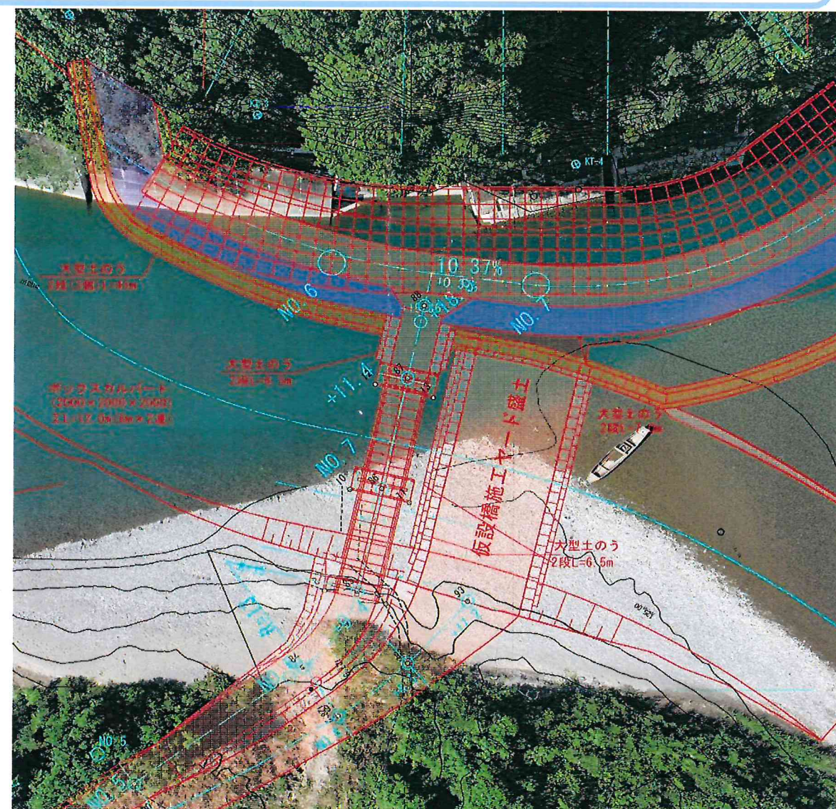
工事用道路(仮橋)設置予定図
