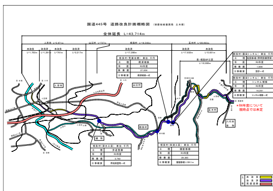
令和3年度 国道445号道路改良計画概略図
