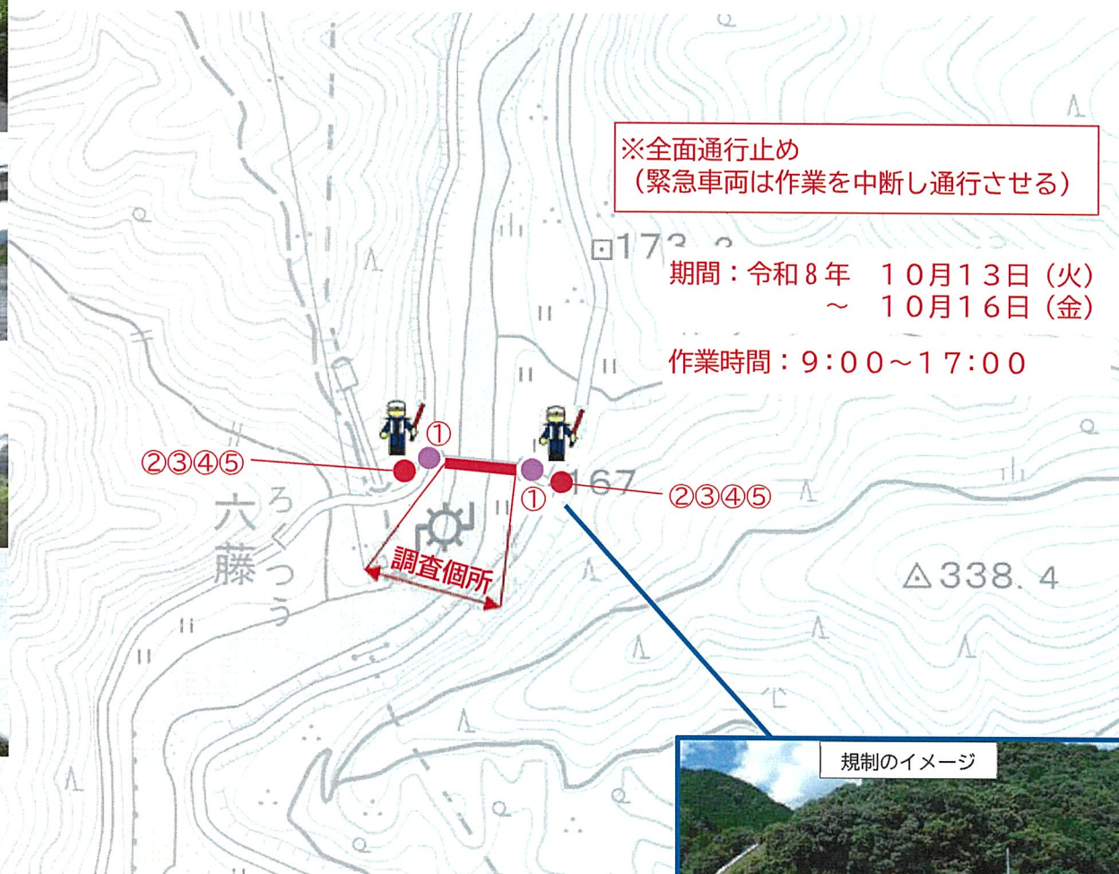
保安対策図：六藤橋（全面通行止め）
